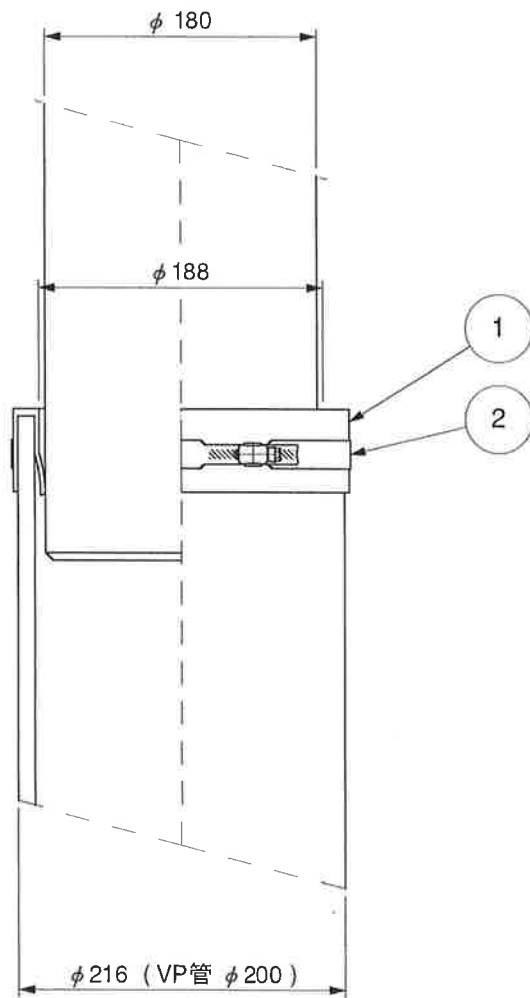
施工状態図
